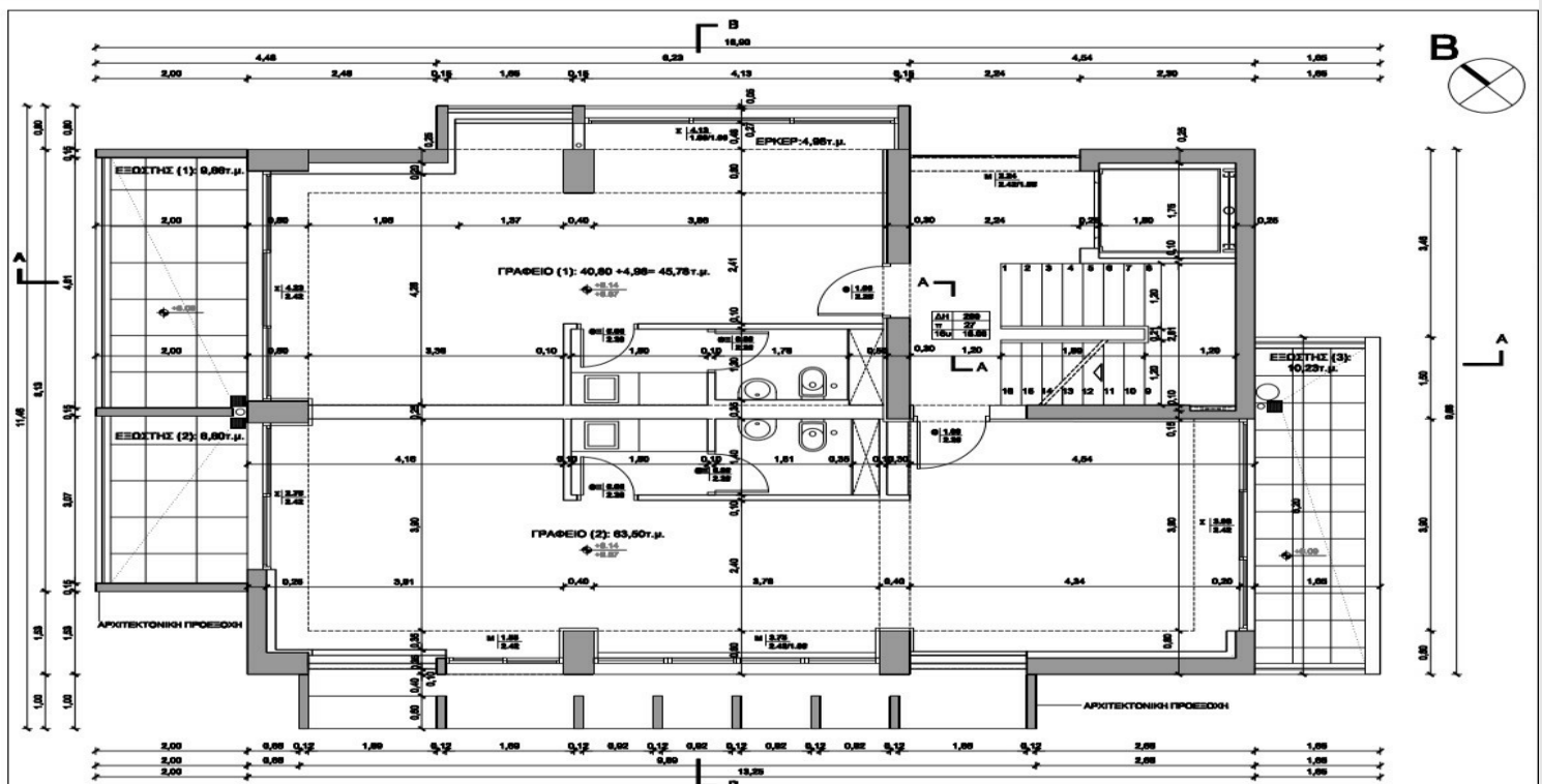
ΤΥΠΙΚΗ ΚΑΤΟΨΗ ΟΡΟΦΟΥ
